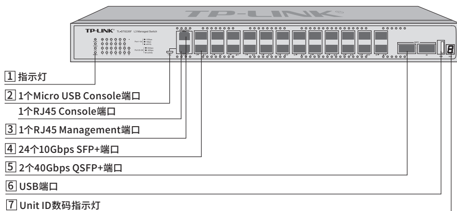
图1-6 TL-ST8226F前面板示意图
