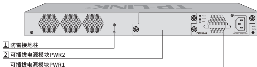
图1-11 TL-ST8226F后面板示意图
