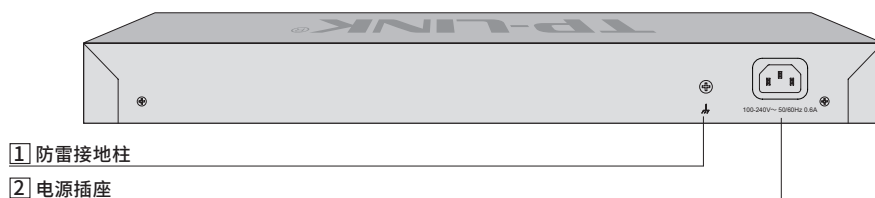
图1-7 TL-SH6428后面板示意图
