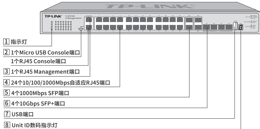
图1-2 TL-SH7428前面板示意图
