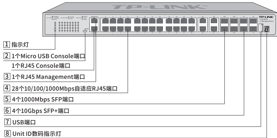
图1-3 TL-SH8434前面板示意图
