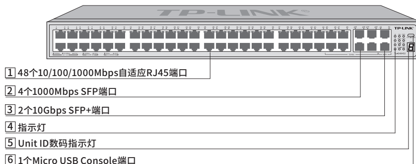
图1-5 TL-SH8452前面板示意图
