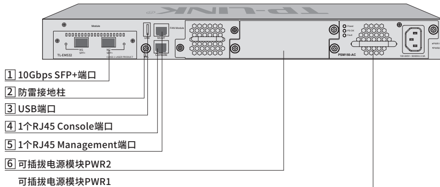
图1-10 TL-SH8452后面板示意图
