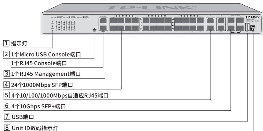
图1-4 TL-SH8434F前面板示意图
